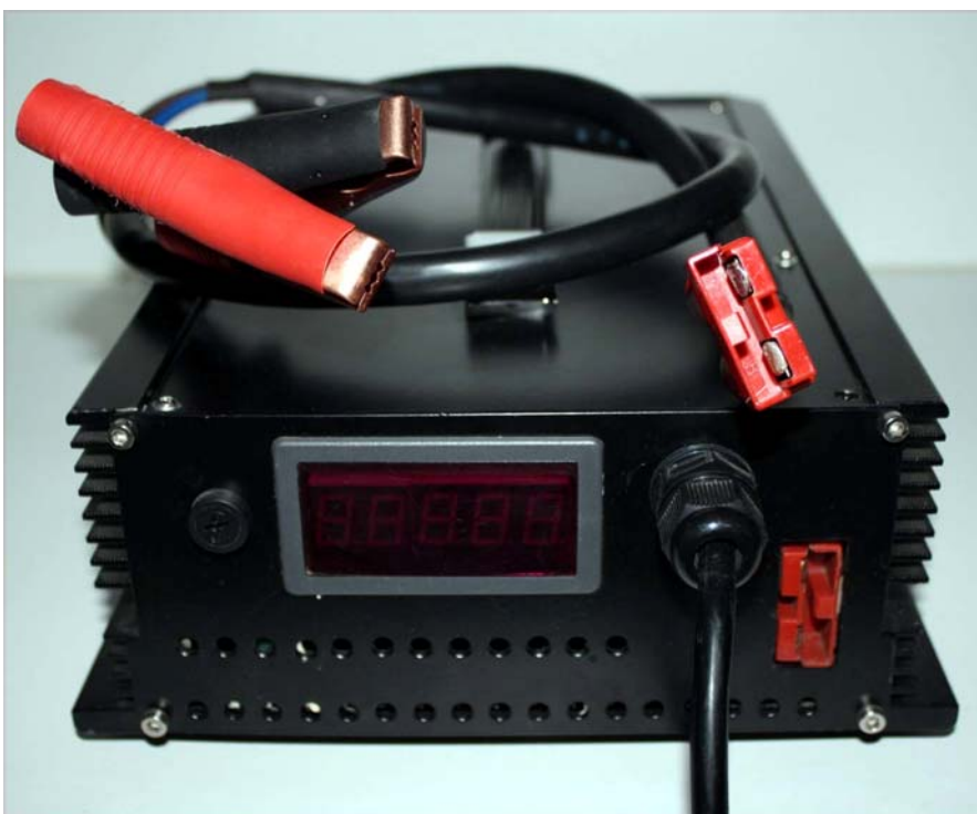
Arrière du Chargeur-Désulfateur – Double ventilation
